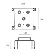
Cassaforma Stoccolma Maxi incasso
