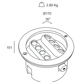
Stoccolma Maxi incasso Carrabile
