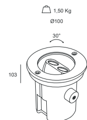
Stoccolma Mini incasso Carrabile
