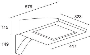
Cairo applique 3,50 Kg
