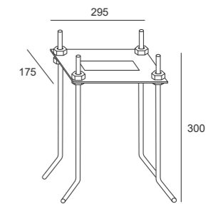
Siviglia piastra tirafondi
