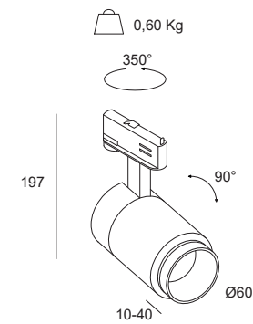
Pippo proiettore da binario
