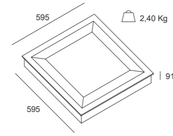
Gundi arretrata incasso
