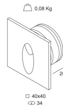
Flash square incasso
